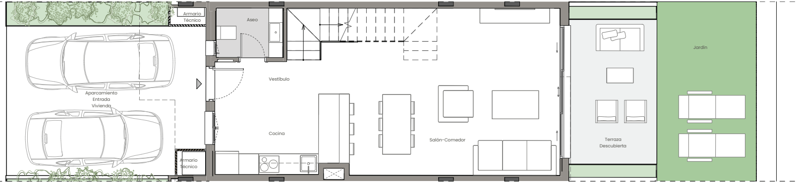
PLANTA BAJA
